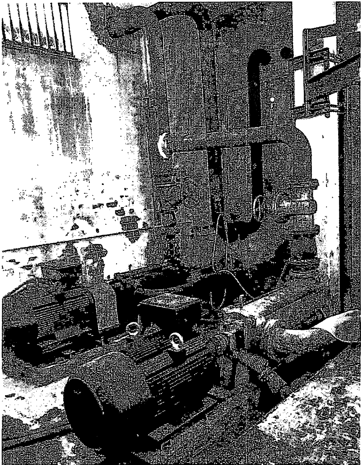
Figura 1 – Centrale Declma Bassa, elettropompa di servizio (destra) e elettropompa di riserva (sinistra)
